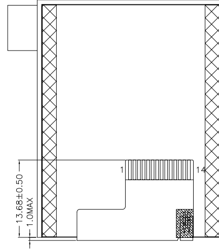
FPC折弯后示图
