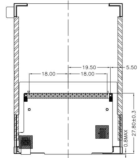
FPC折弯后示意图
